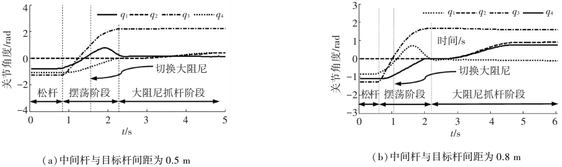
图 8 中间杆与目标杆间距分别为 0.5 m 和 0.8 m 时各关节角度曲线
