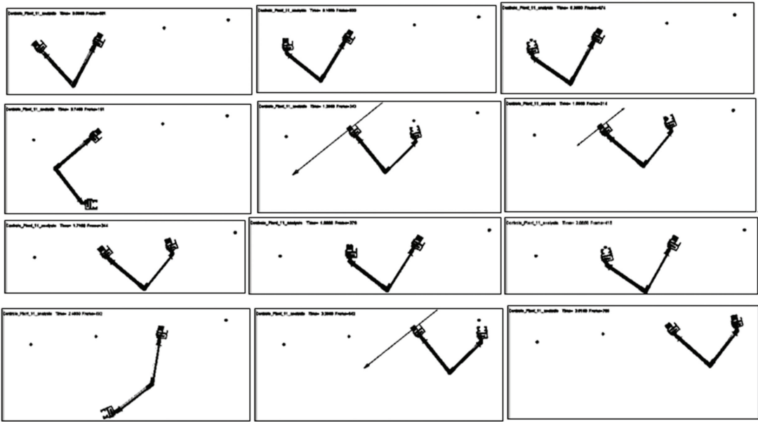
图 5 仿猿双臂手机机器人连续移动仿真视频截图
