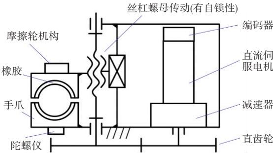
图 3 机器人手爪结构简图
