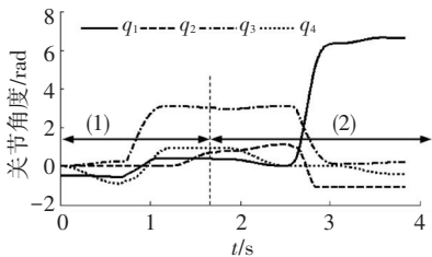
图 6 连续移动仿真各关节轨迹
