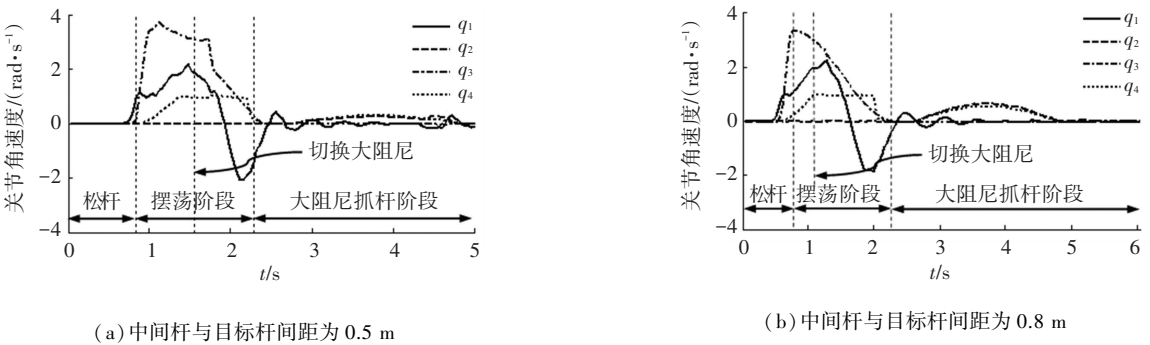
图 9 中间杆与目标杆间距分别为 0.5 m 和 0.8 m 时的关节角速度曲线
