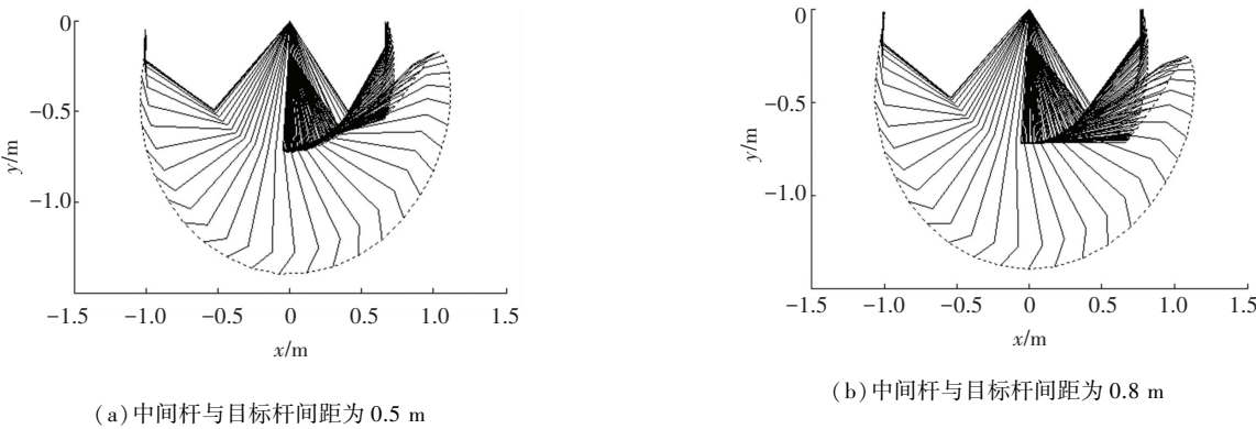
图 7 中间杆与目标杆间距分别为 0.5 m 和 0.8 m 时的机器人运动轨迹
