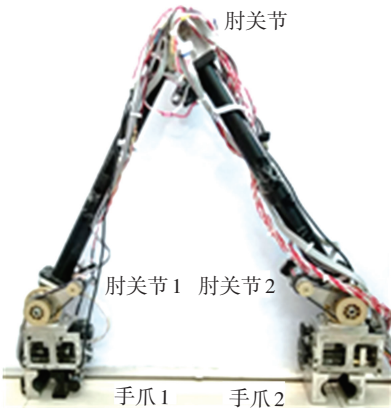
图 1 BARDAH-I 型仿猿双臂手机机器人
