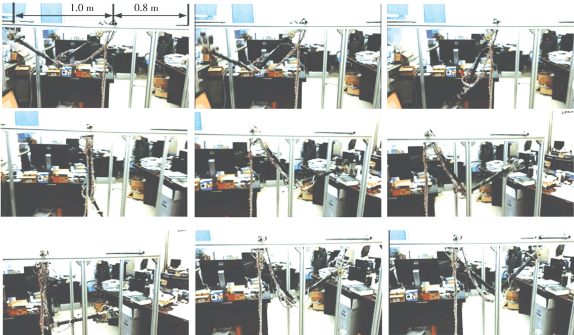
图 11 中间杆与目标杆间距为 0.8 m 时机器人摆荡抓杆控制实验视频截图
