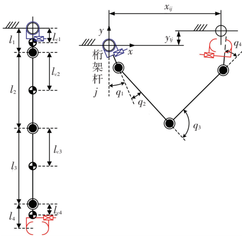
图 2 机器人杆件参数示意
