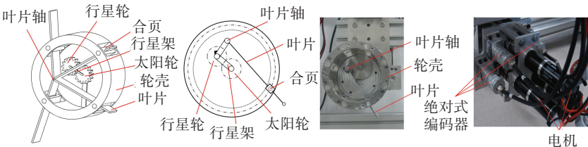
图 1 可动叶片车轮机构 [19]
