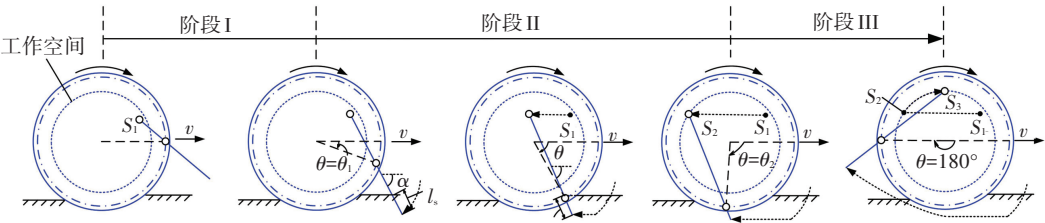
图 2 车轮从 0° 旋转到 180° 时,ALW-土壤一个完整交互作用过程中的叶片轨迹
