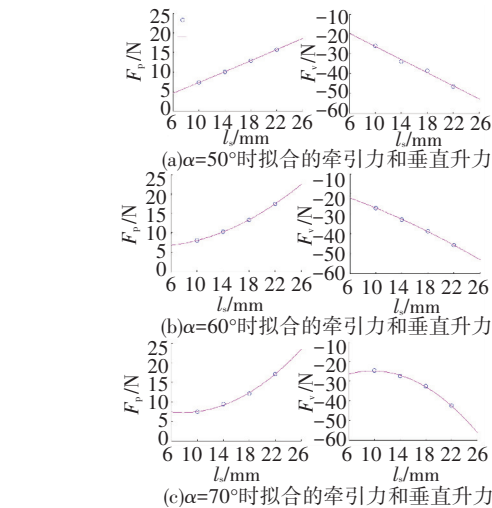
图 11 倾斜角度 \alpha 为 50^\circ , 60^\circ , 70^\circ 时,根据公式(3)、(4)拟合的牵引力(左列)和垂直升力(右列)
