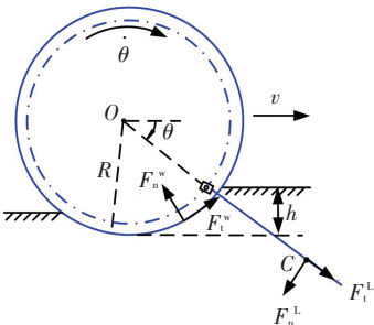
图 3 ALW-土壤交互作用力学模型
