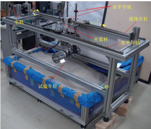
图 5 ALW-土壤交互作用测试平台 Fig.5 ALW-soil interaction testbed
