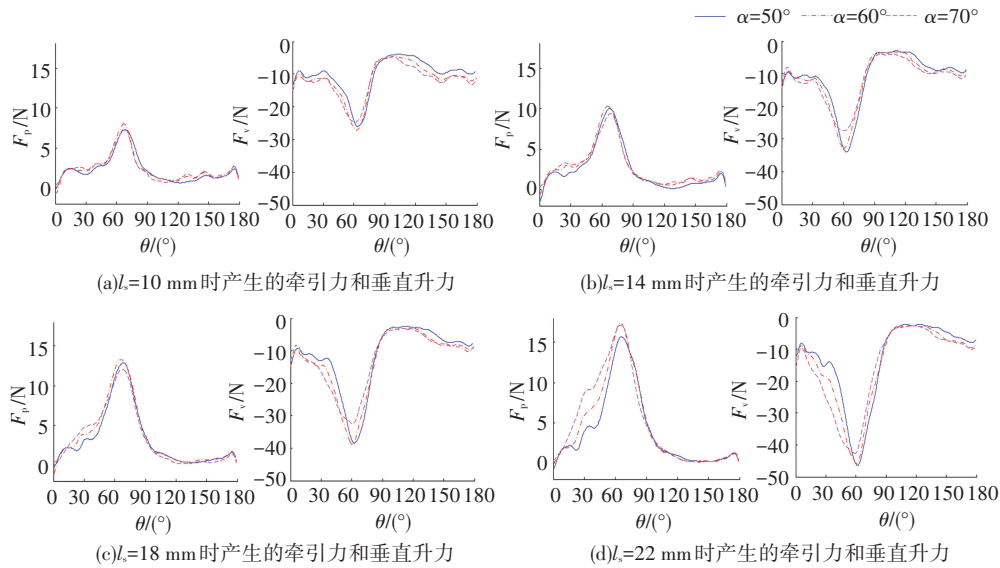
图 10 沉陷长度为 10,14,18 和 22 mm 时,产生的牵引力(左列)和垂直升力(右列)
