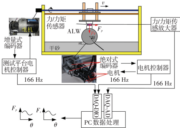
图 6 数据采集系统 Fig.6 Data acquisition
