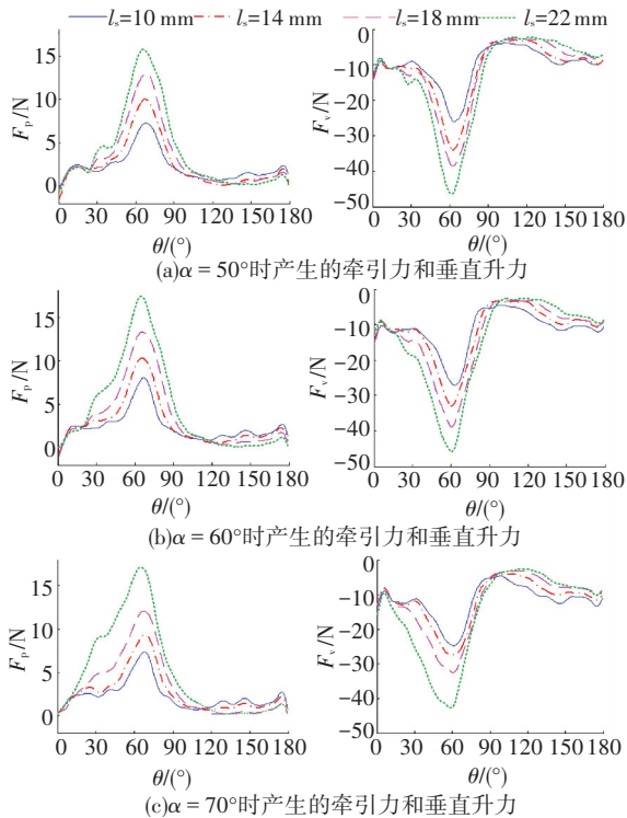
图 9 倾斜角度为 50^{\circ}, 60^{\circ} 和 70^{\circ} 时,产生的牵引力(左列)和垂直升力(右列)
